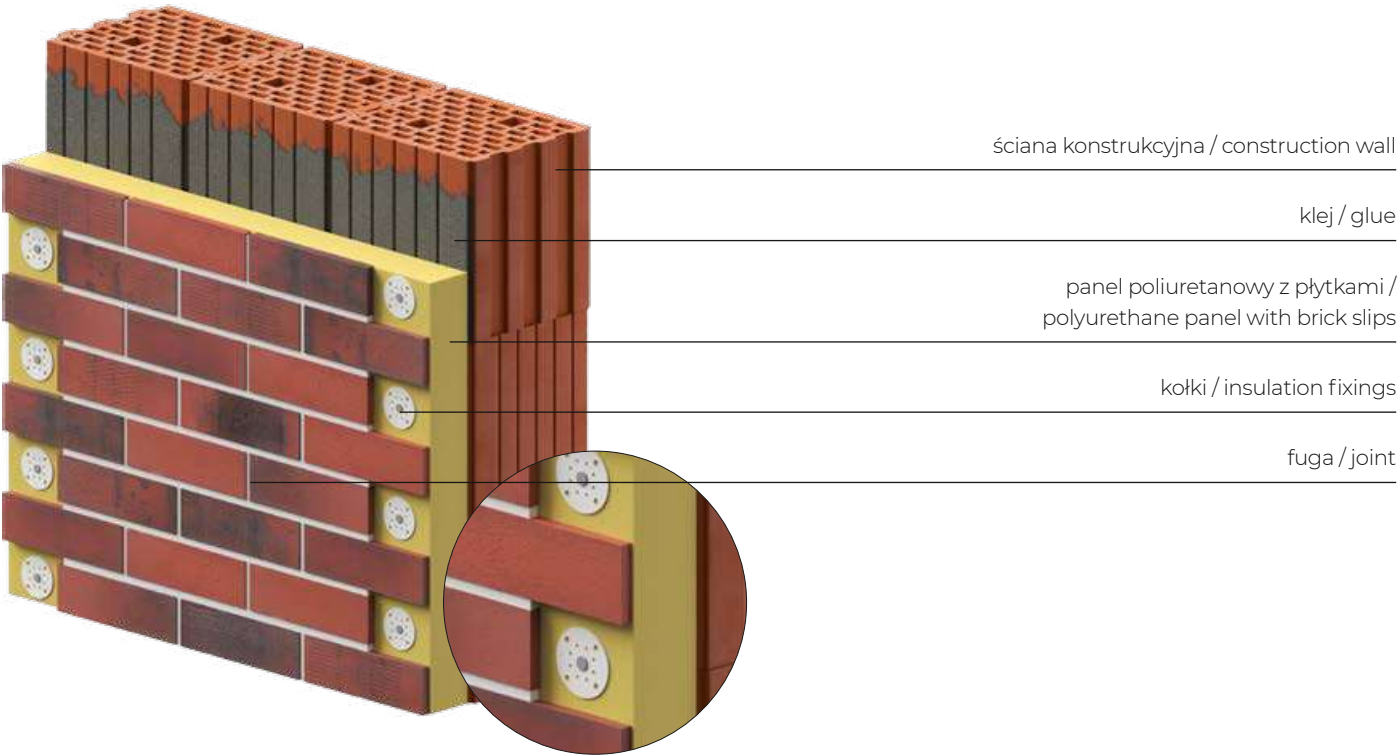
System z płytkami zatopionymi w poliuretanie / System with brick slips embedded in polyurethane
