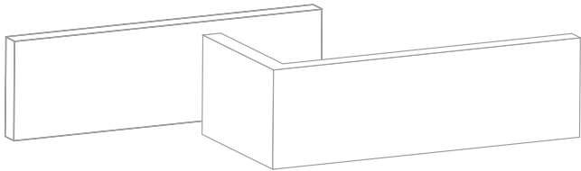
Płytką elewacyjną Brick slip NF - 71 x 240 x 14 mm
