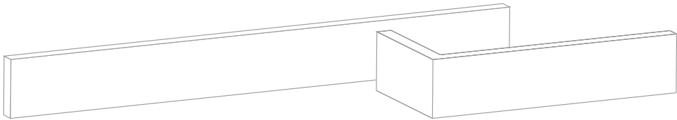
Płytką elewacyjną Brick slip LF - 52 x 490 x 14 mm
