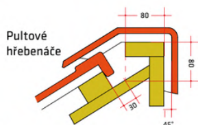
Řez střešním pláštěm.
